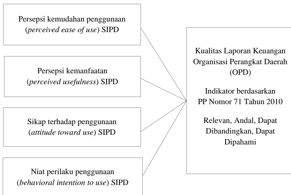
Gambar 2.5 Kerangka Pemikiran
